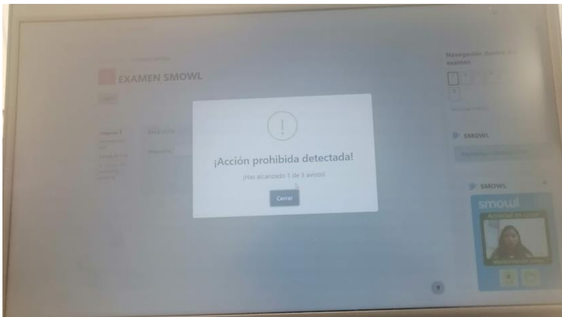
Ilustración 15 Advertencias Smowl
