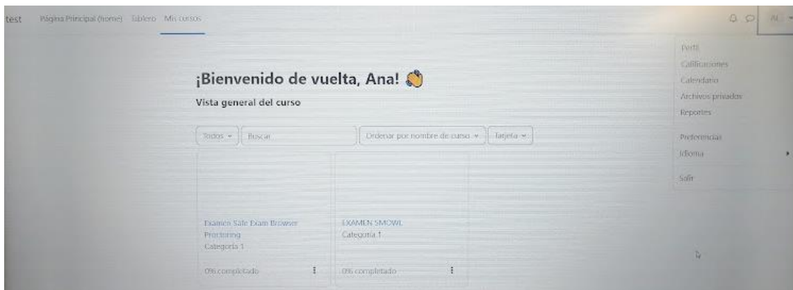
Ilustración 4 Clases
