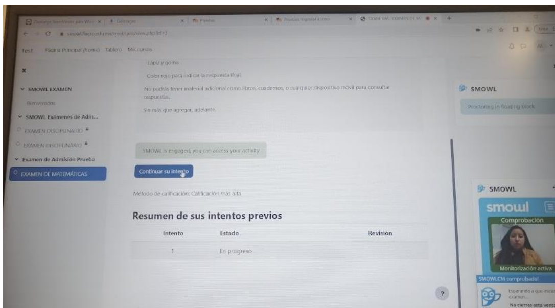
Ilustración 13 Monitorización activa
