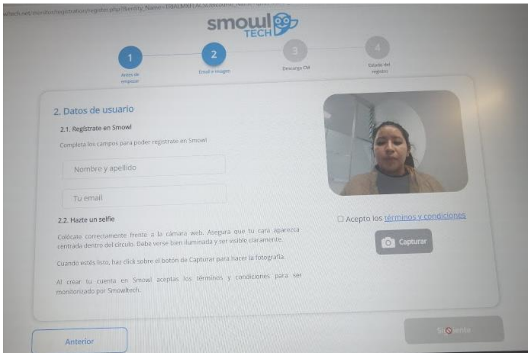
Ilustración 12 Registro Paso 2
